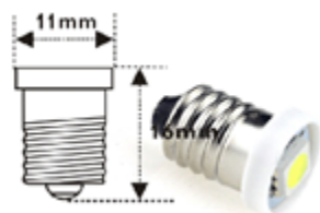
E10 1w (varmvit) 6 volt
