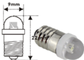
E10 0,5w (varmvit) 6 volt
