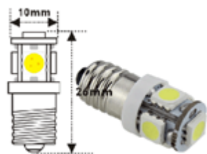
E10 1,5w (varmvit) 6 volt
