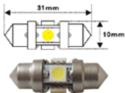
Spollampa 1,5w (varmvit) 31mm 6 volt
